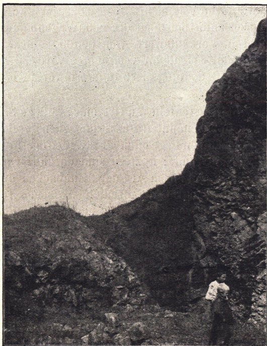
Einlagerung von Tuff zwischen Basalt. Kleiner Kulm.
