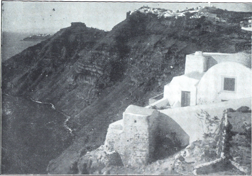
Der Steilabsturz der Insel Thera.
