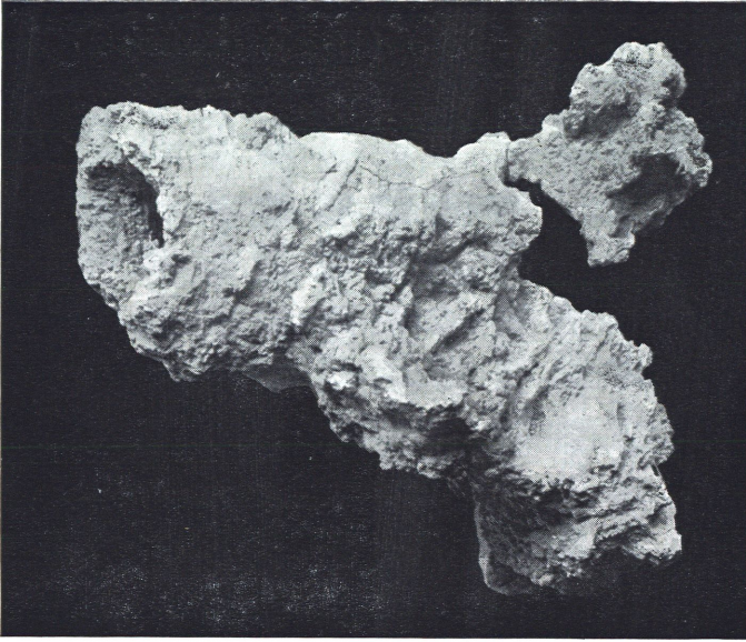
Geyser Röhre aus Kieselginter.
