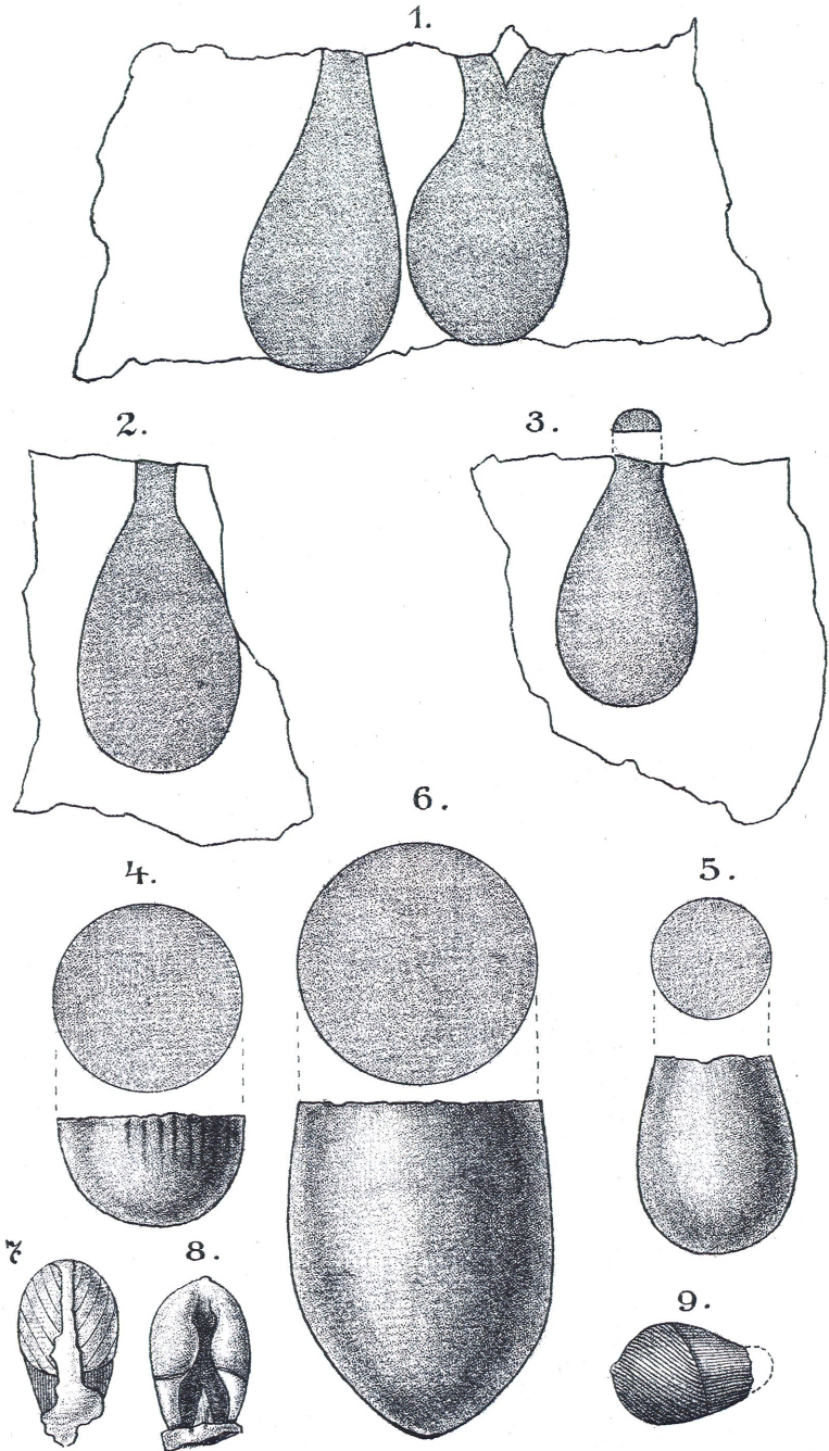
Fig. 1. 2. 3. Bohrlöcher im Jurakalk. Fig. 4. 5. 6. Cenomane Ausfüllung von Bohrlöchern. Fig. 7. 8. 9. Pholas rugosa . Fig. 7 zeigt Teile der Hülle.
